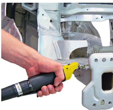
Système de démontage vitres voitures et camions
