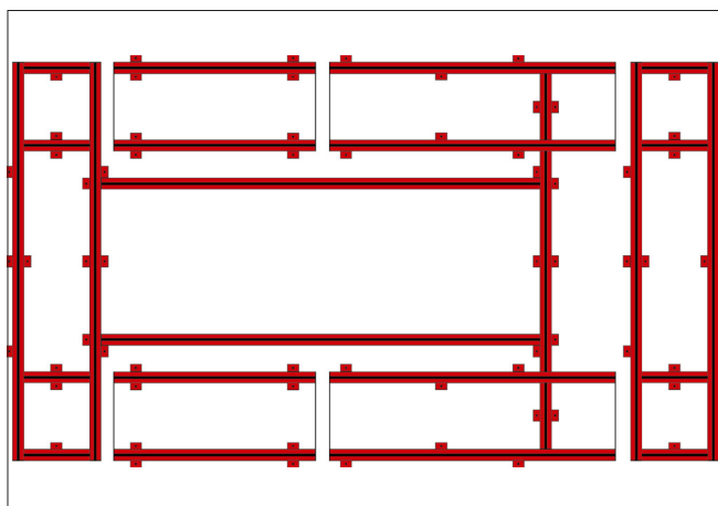
ASK1605901PLS - châssis 4 x 6,52 m
