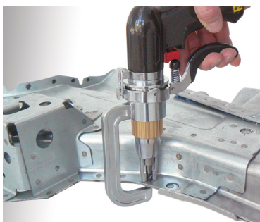
Foreuse pour points de soudure - Vario Drill WS90
