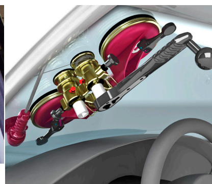
Système de démontage vitres voitures et camions
